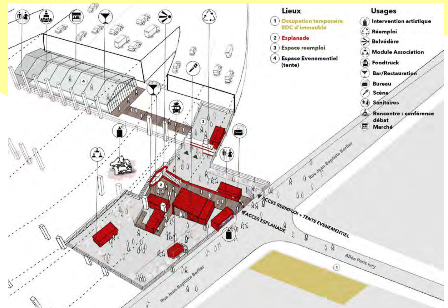
Axonométrie des aménagements de l'esplanade sous le périphérique. Crédits : Palabres Architectes.
